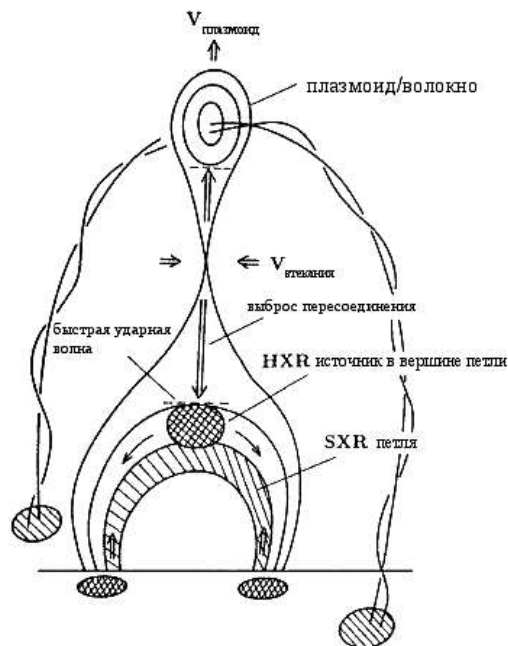
Рис. 2. Унифицированная модель солнечной вспышки, основанная на механизме магнитного пересоединения с выбросом плазмоида. HXR – источник жесткого рентгеновского излучения; SXR – источник эмиссии в мягкой рентгеновской области спектра [Shibata, 1998].
